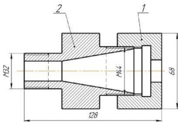
1 – Корпус; 2 – Штуцер
